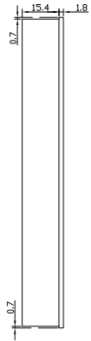
侧面图
