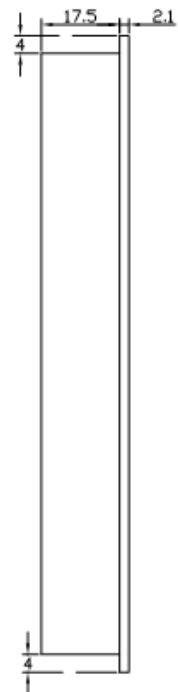
侧面图
