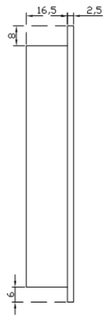
侧面图
