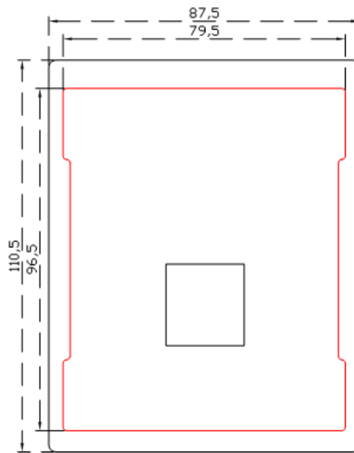
正面图
