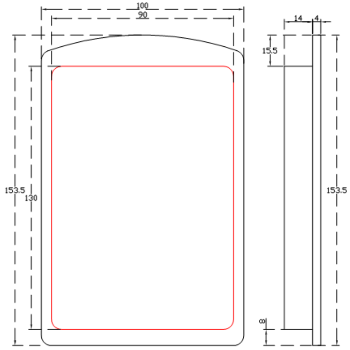
正面图
