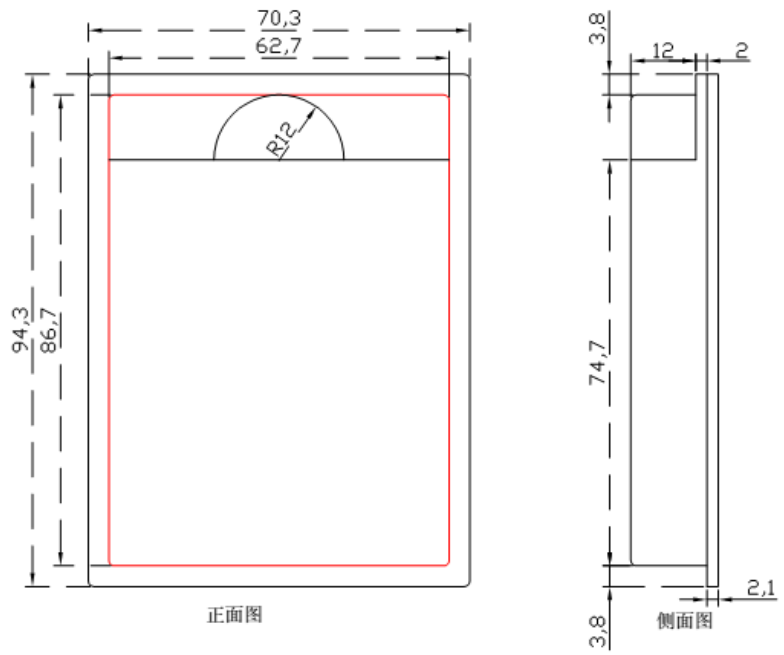
正面图
