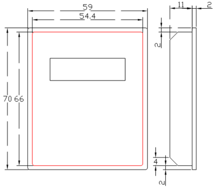
侧面图
